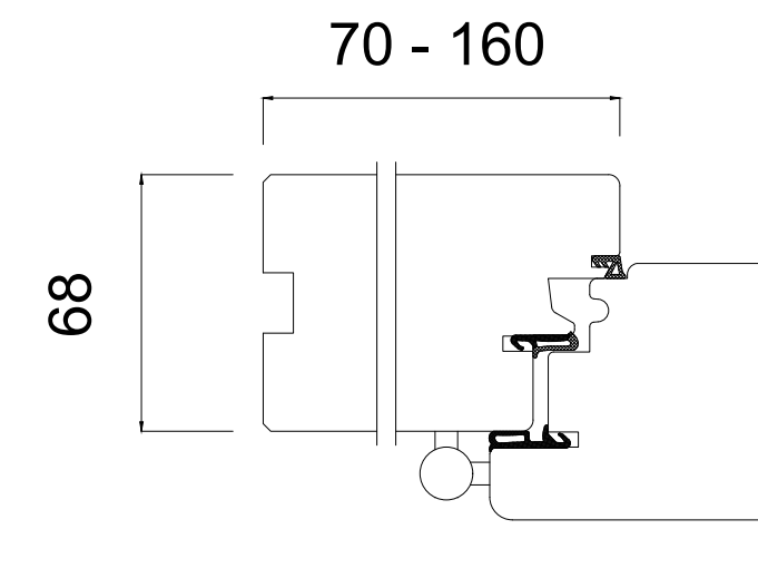
Telaio allargato fino a 160 mm Altre misure a richiesta
